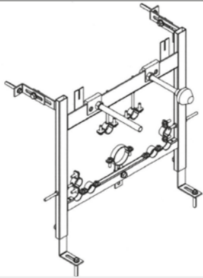
Staffa metallica per il montaggio del bidet alla parete 65.00 €
