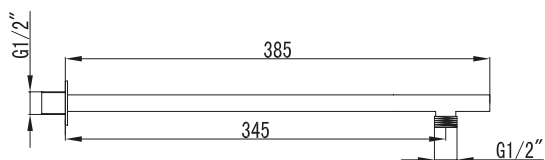
Bras mural carré en laiton
