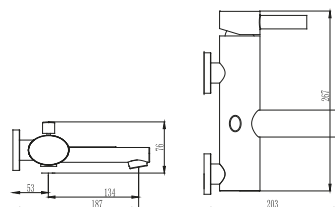
Mitigeur de baignoire 199.00 €
