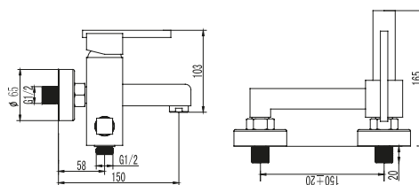
Mitigeur de baignoire 179.00 €
