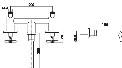
Mitigeur lavabo mural
