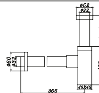
Siphon en laiton tubulaire 1/4 avec bouchon de dégorgement
