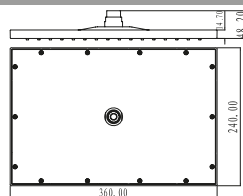
Pomme de Pomme de tête carré ABS 24x36cm 59.00 €
