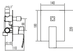
Mitigeur de douche inverseur 2 voies
