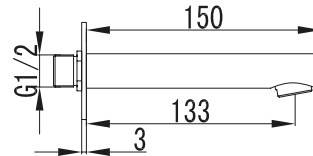
Bec mural en laiton 13 cm
