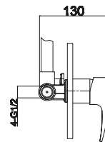
Mitigeur de douche monocommande Mécanisme céramique
