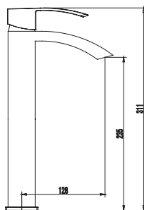
Mitigeur lavabo rehaussé. 199.00 €
