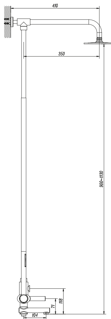
Combiné de douche 449.00 €
