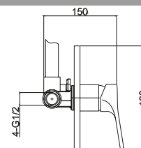
Mitigeur de douche monocommande 59.00 € Mécanisme céramique
